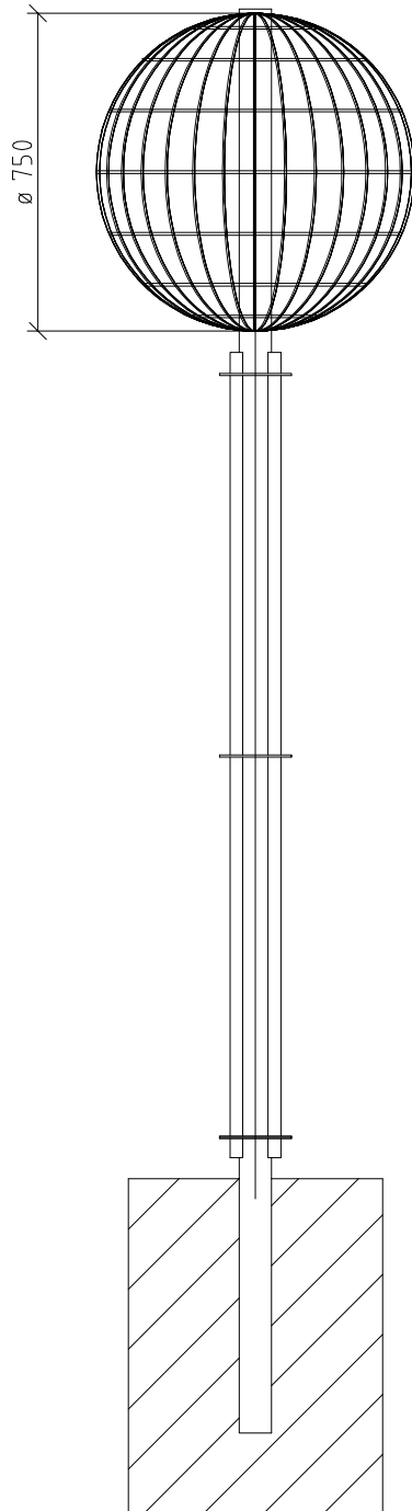
Rankbaumkugel Typ I Stütze Ambiente L=1800mm Kugel \varnothing 750
