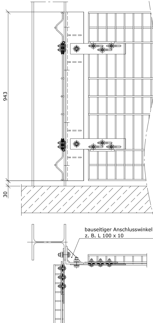
Anschlussdetail Stützenverdrehung (schraubbar) bauseitige und statisch ausreichend dimensionierte Anschlusswinkel
