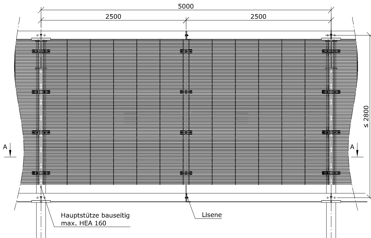
Fassadenausschnitt LINEAR Standardraster = 5000 mm
