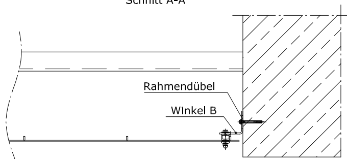
Schnitt A-A
