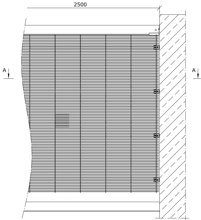
Fassadenausschnitt LINEAR Betonanschluss
